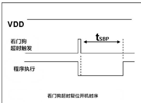
图 10: 看门狗超时溢出时序图
