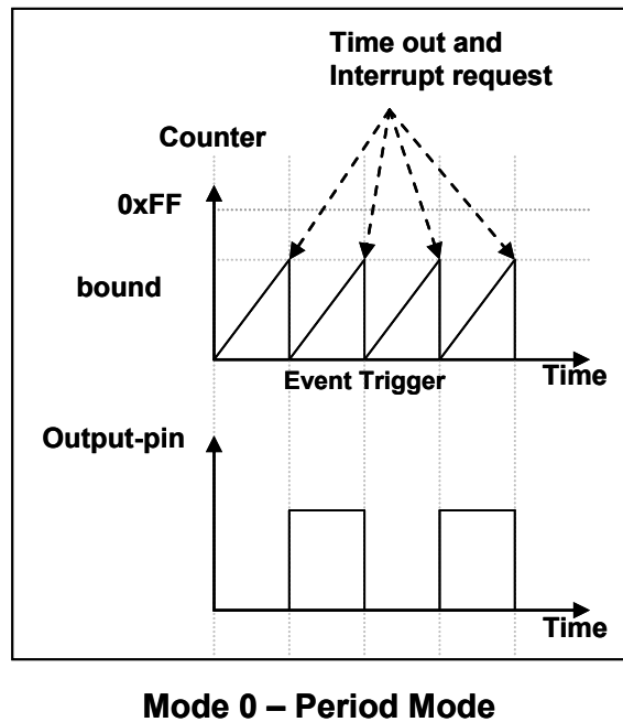
图 16: Timer3 周期模式的时序图
