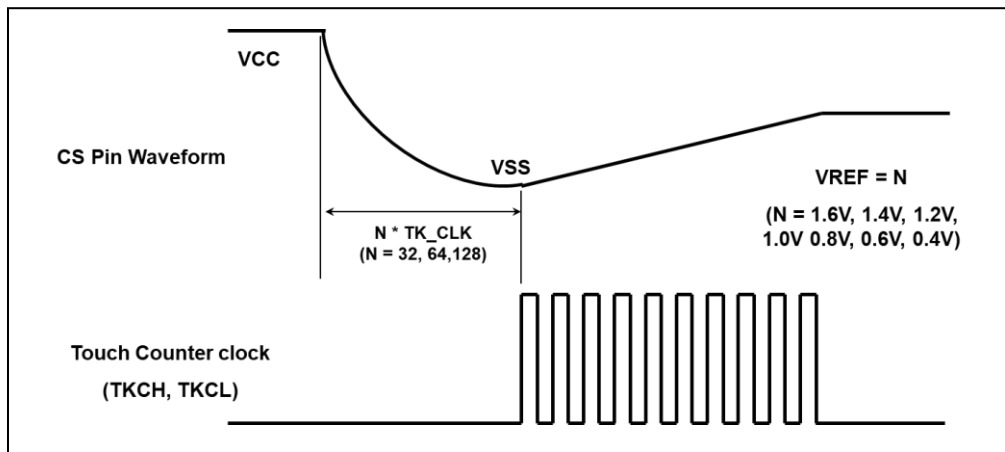
图 18: 触摸转换的时序图
