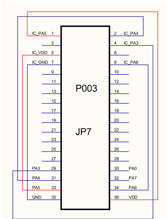
图 21: 使用 P003 时，PMS161-S08B JP7 跳线原理图
