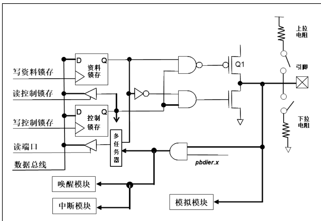
图 12: IO 引脚缓冲区硬件图
