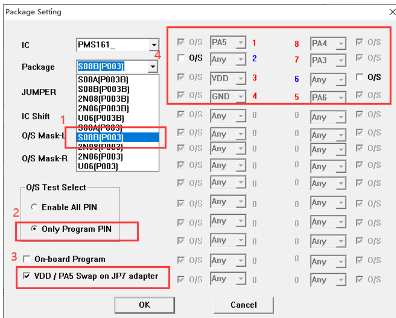
图 20: PMS161-S08B 在 P003 转档配置
